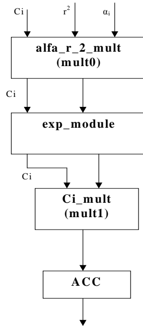
Fig. 1. EP module block diagram
